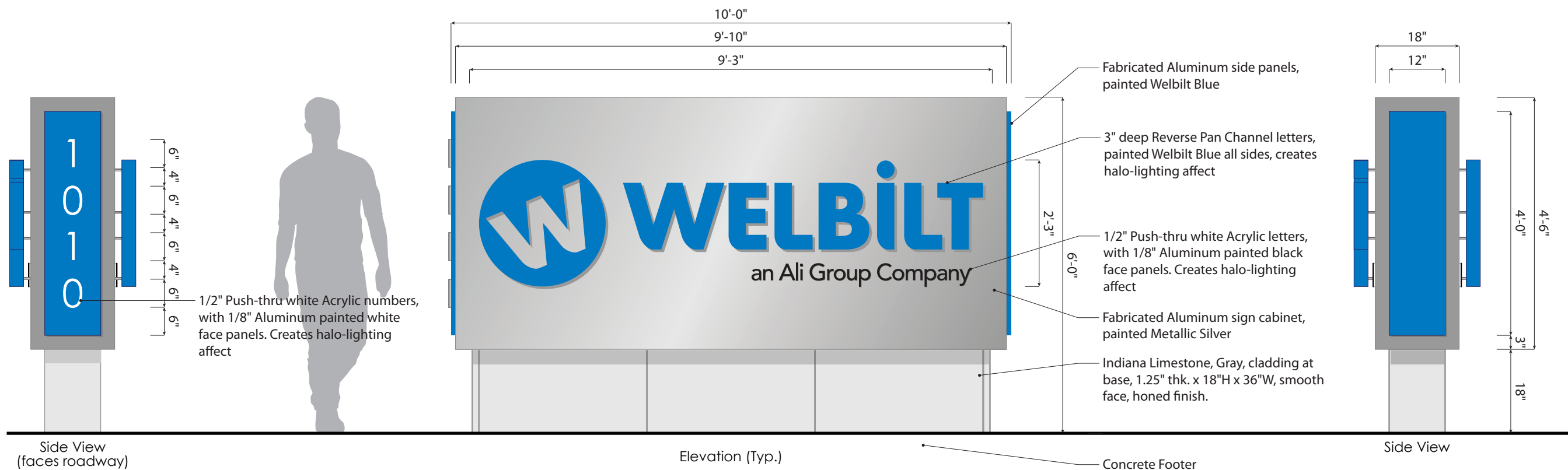
Monument Sign Scale: 1/2" = 1' - 0"
