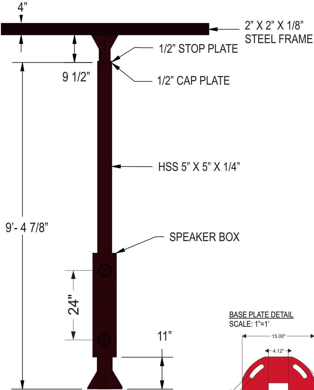
FRONT VIEW SCALE: 1:20
