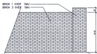
06 Screen Wall Elevation Scale: 3/8" = 1'-0"
